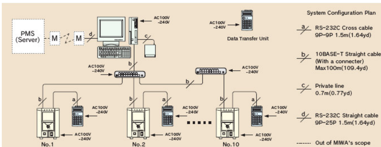
Przykładowa konfiguracja urządzeń (wersja KME)
